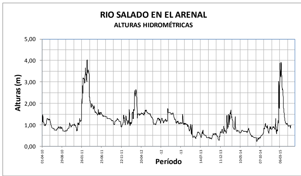
Alturas Hidrométricas pertenecientes a la BDI de la SSRHN – Período 01/04/2010 – 31/05/2015
