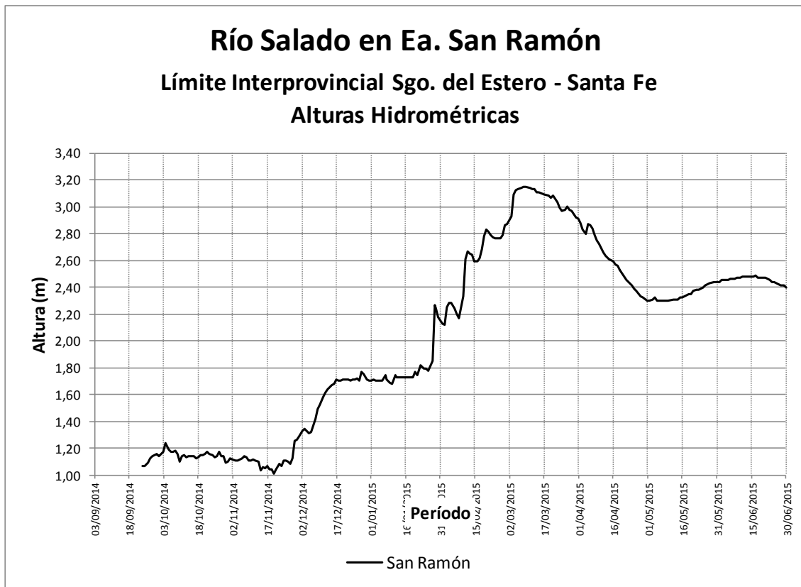
Los datos corresponden al sensor de presión, período 24/09/2014 – 30/06/2015.
