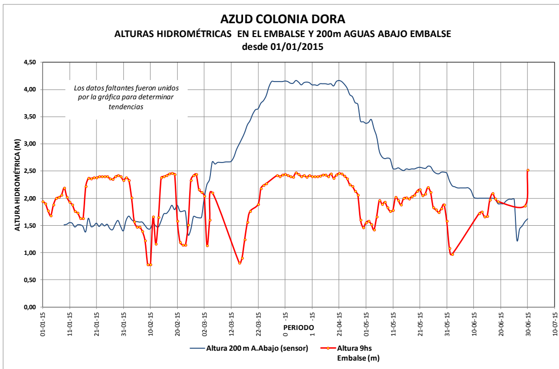
Alturas hidrométricas correspondientes al período 01/01/2015 – 30/06/2015.
