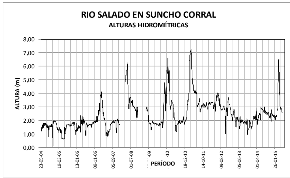
Alturas Hidrométricas pertenecientes a la BDI de la SSRHN – Período 30/05/2004 – 30/05/2015
