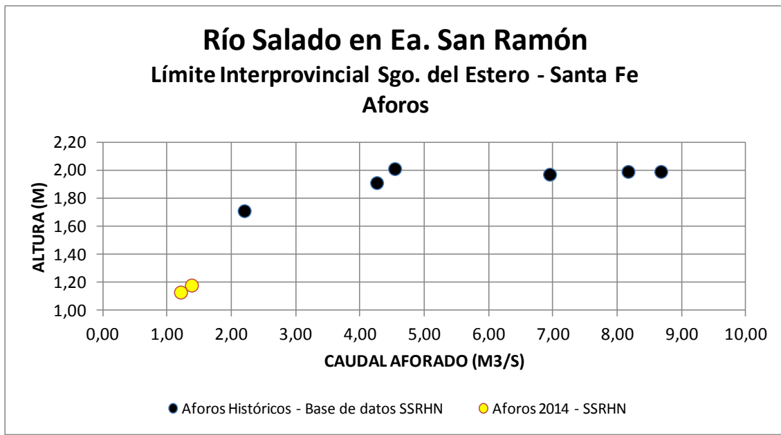
Los aforos históricos corresponden a la Base de Datos Hidrológica Integrada (BDHI) de la Subsecretaría de Recursos Hídricos, período 2010/2011. En Amarillo aforos de Setiembre de 2014.
