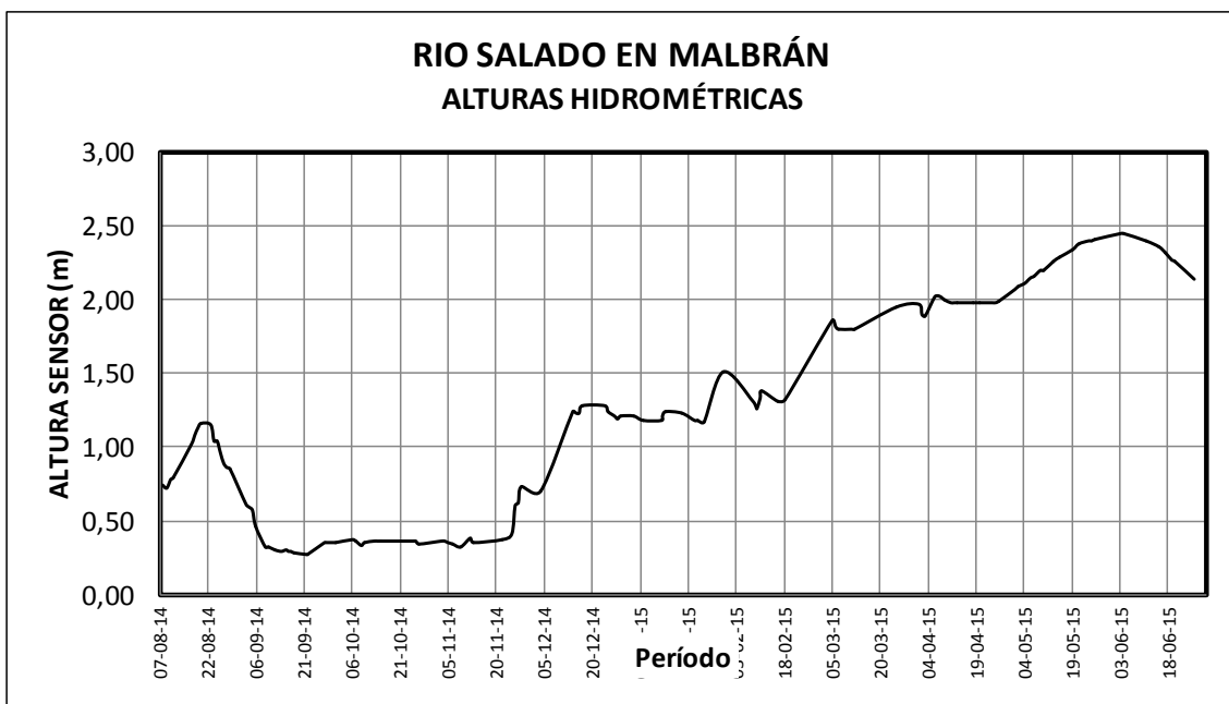
Alturas registradas por el sensor. Período 08/08/2014 al 30/06/2015. La línea une datos consecutivos y no consecutivos ( por ausencia de datos), para visualizar tendencia.
