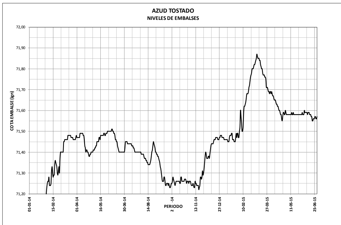
En este gráfico vemos las variaciones en los niveles del embalse, correspondientes al periodo 01/01/2014 – 30/06/2015.
