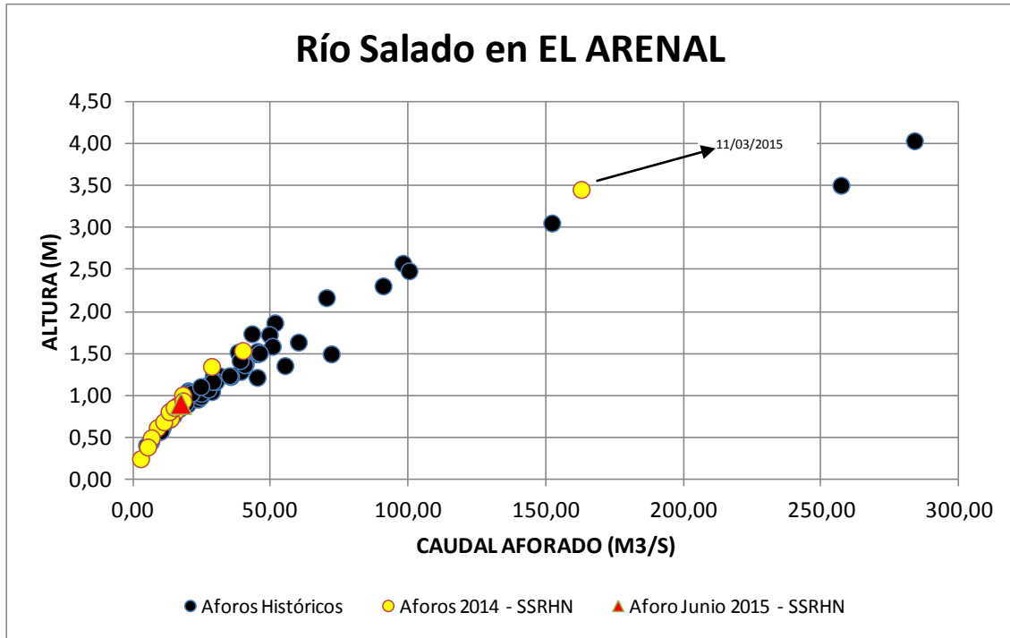
Los aforos históricos corresponden a la Base de Datos Hidrológica Integrada (BDHI) de la Subsecretaría de Recursos Hídricos, período 2010/2013. En amarillo aforos período 2014/15. En rojo el aforo de Junio de 2015.
