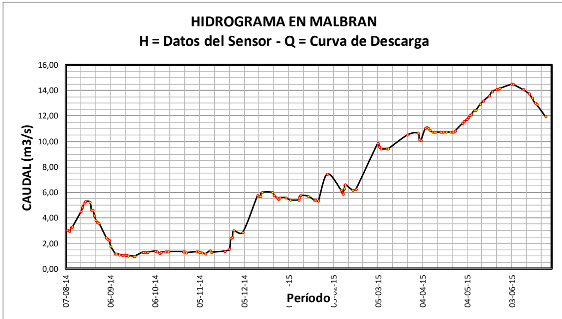
Gráfico de alturas registradas por el sensor y caudales calculados por la curva de descarga. Se presenta el período 08/08/2014 al 30/06/2015. La línea une datos consecutivos y no consecutivos( por ausencia de datos), para visualizar tendencia.
