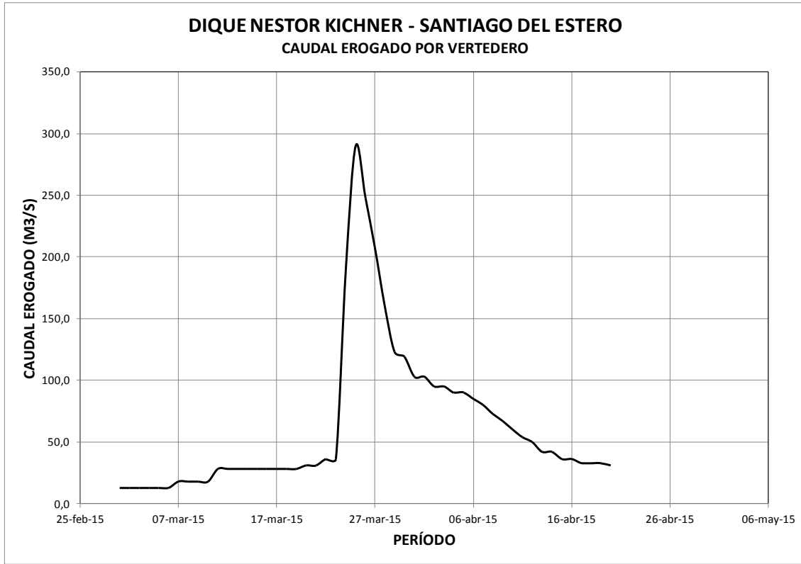
Caudal erogado por vertedero. Período 01/03/2015 – 20/04/2015
