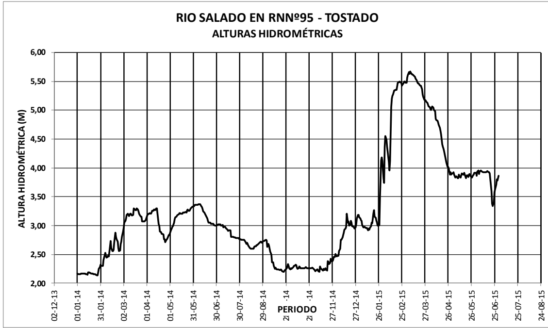
Alturas Hidrométricas período 01/01/2014 – 30/06/2015
