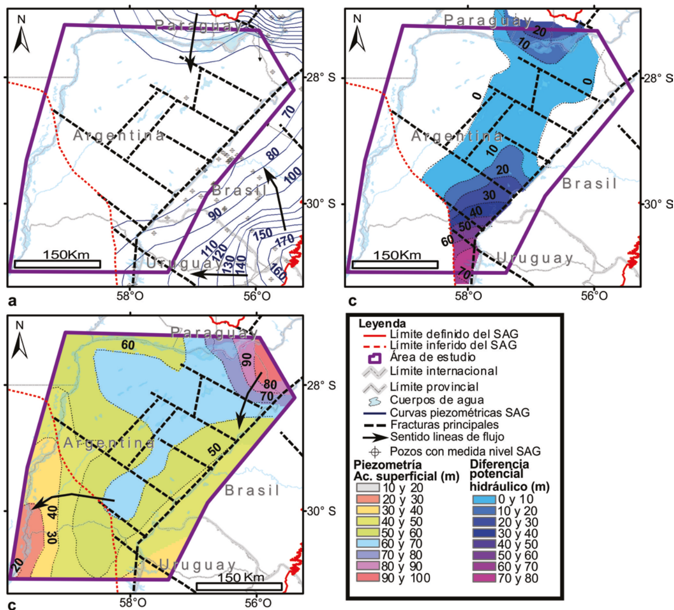
Figura 8: a) Mapa piezométrico del Sistema Acuífero Guaraní (SAG); b) Mapa piezométrico del acuífero superior y; c) Diferencia de potencial hidráulico entre ambos. Modificado de Nittman (2014).
