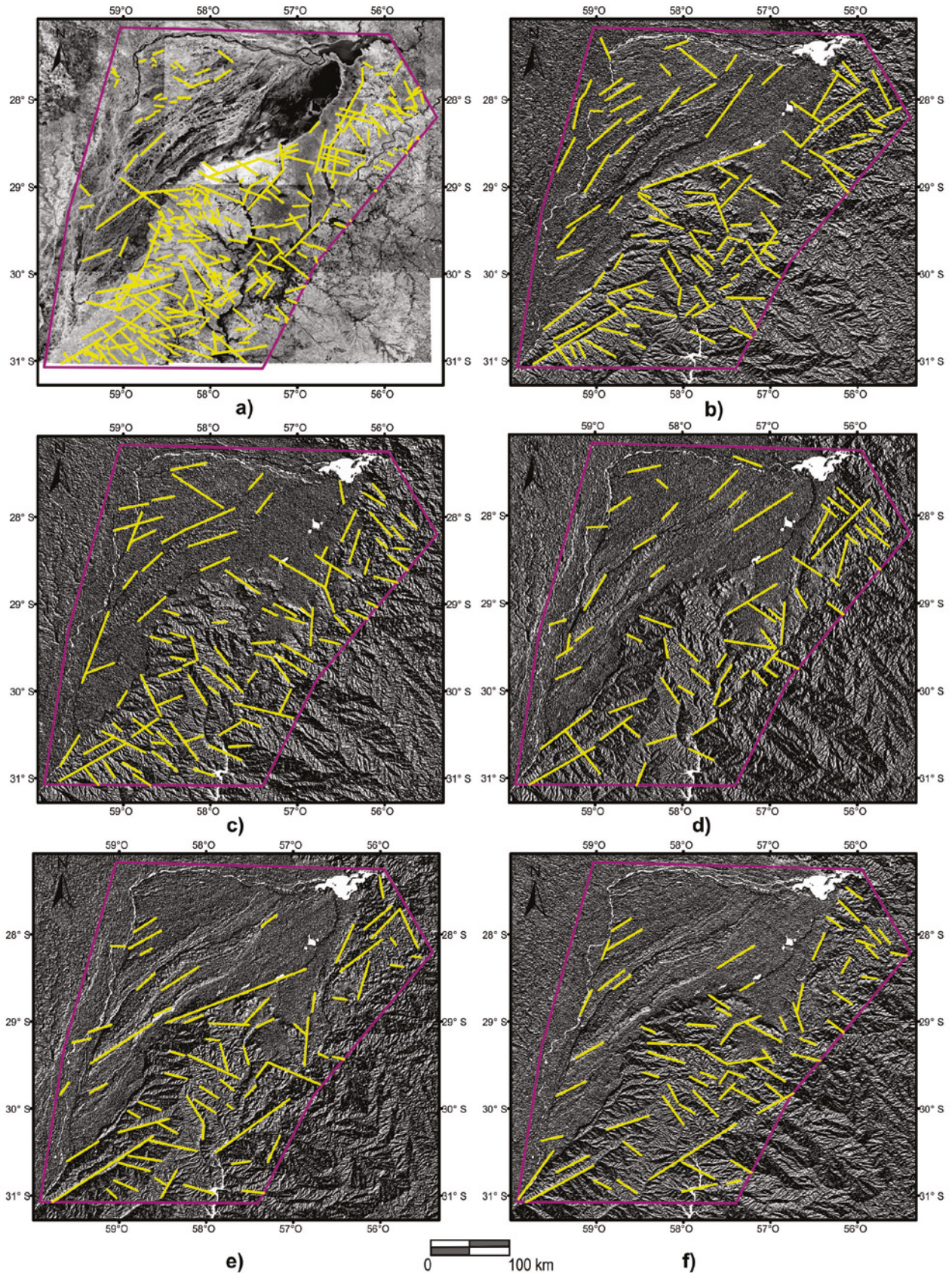
Figura 6: a) Lineamientos medidos en imagen Landsat-ETM; b-f) Lineamientos medidos en modelo digital de elevación con orientación de la iluminación desde la dirección acimutal 0° (b), 45° (c), 90° (d), 135° (e) y 180° (f).
