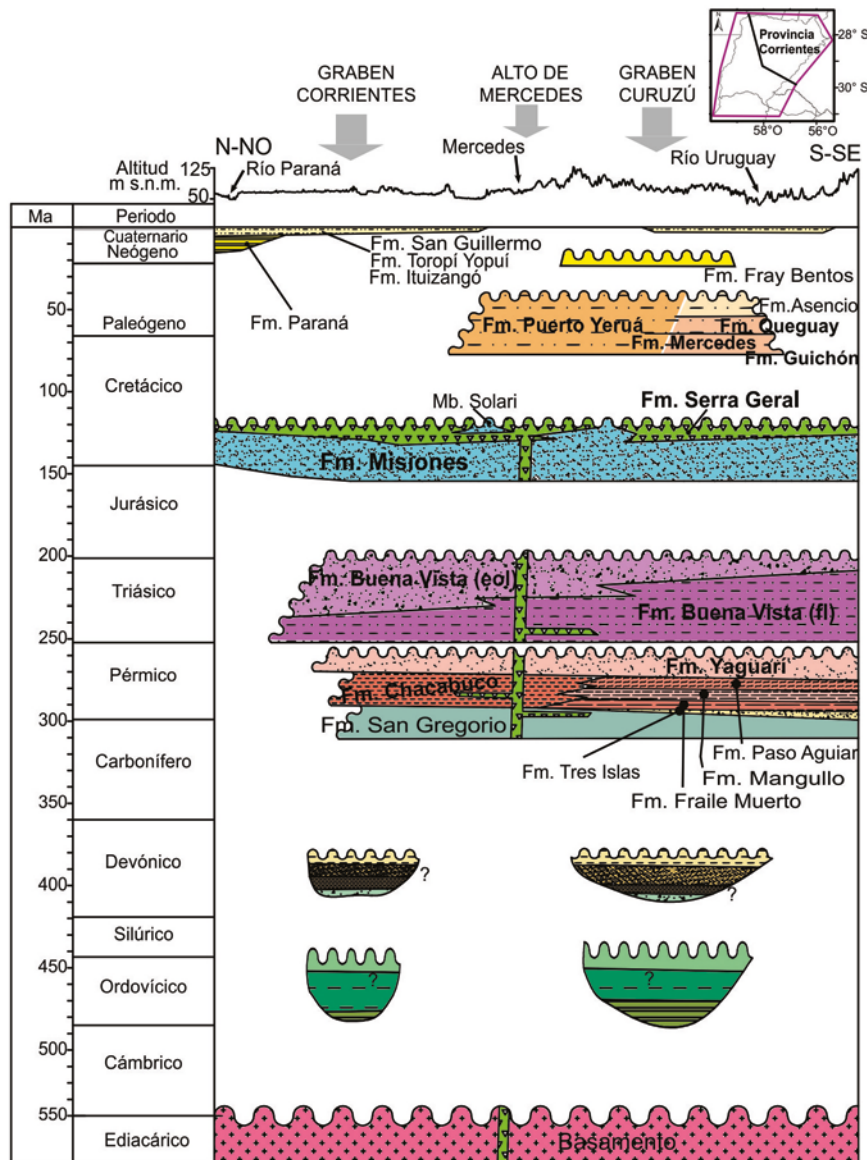
Figura 3: Columna estratigráfica propuesta para Corrientes según Mira et al. (2015).
