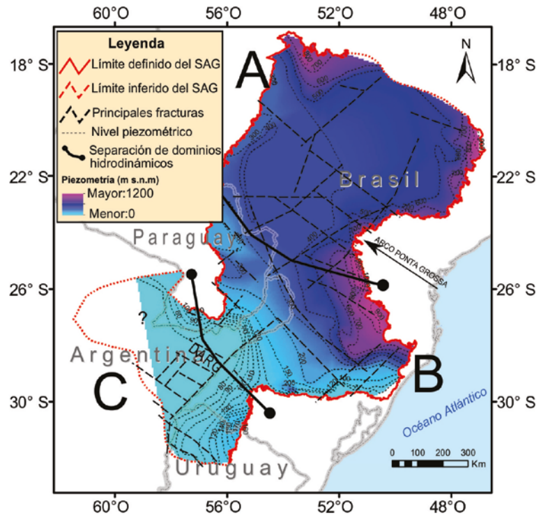
Figura 1: Mapa piezométrico del Sistema Acuífero Guaraní (SAG) (modificado de Mira (2012) y Nittmann (2014) que incluye las principales fracturas en la cuenca de Paraná (según Soares 2008). Se muestra la división en tres zonas según el comportamiento hidrodinámico.
