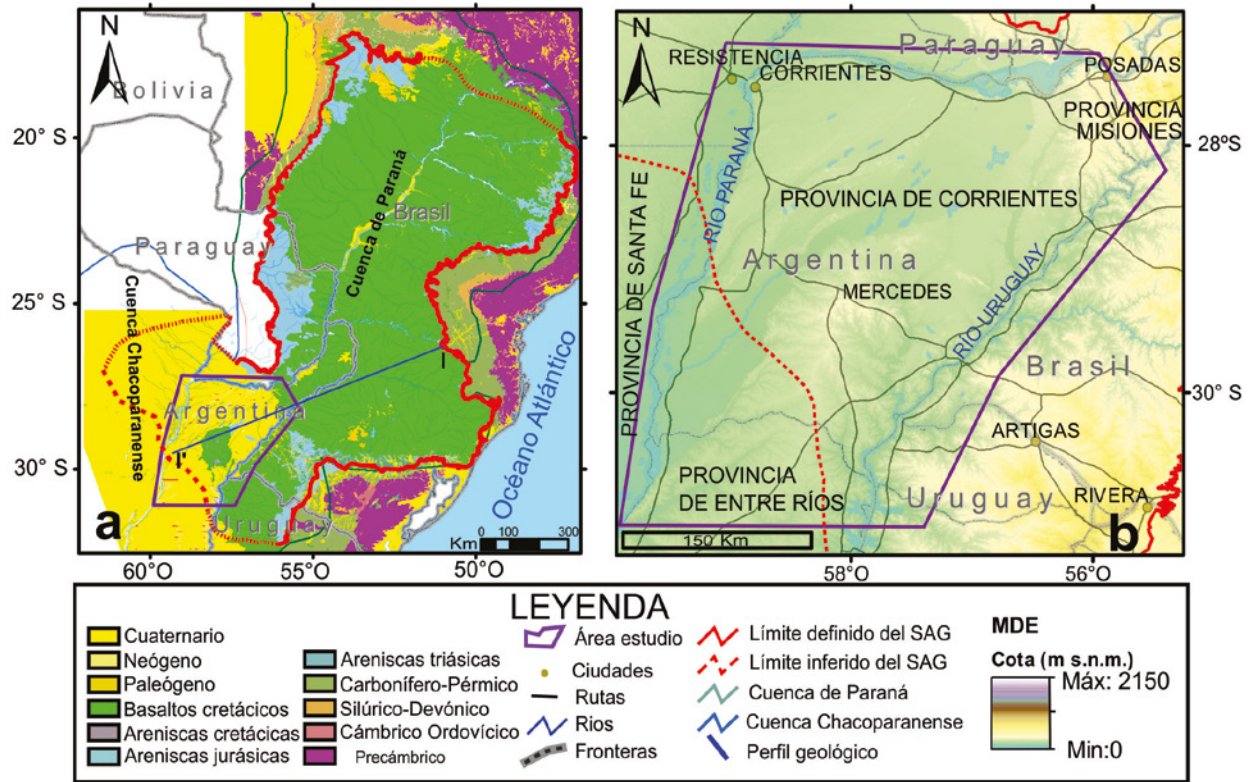
Figura 2: Mapa de ubicación del área de estudio (a) y modelo digital de elevación (b). A la izquierda se muestra un esquema geológico regional (modificado de Achilli et al. 1998, Bossi y Ferrando 2001, Schobbenhaus y Bellizzia 2001 y Almeida et al. 2004), incluyendo las principales litologías y la extensión de las cuencas de Paraná y Chacoparanense.
