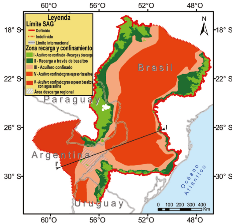
Figura 9: Zonificación de la recarga para el Sistema Acuífero Guaraní (SAG) en función del espesor de los basaltos que confinan el acuífero y de la densidad de lineamientos en la zona de Corrientes. Elaboración propia a partir de los datos de espesores de Foster et al. (2009) y Mira et al. (2015).
