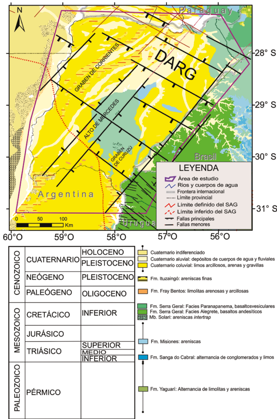
Figura 4: Mapa geológico y tectónico del área de estudio.
