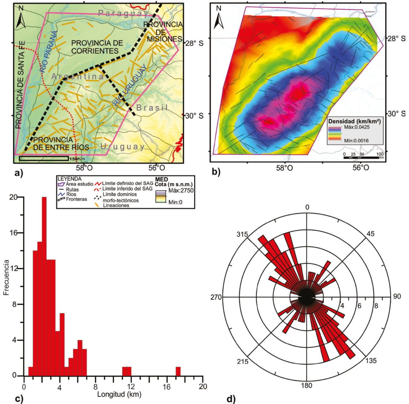
Figura 7: a) Mapa resultado de lineaciones medidas en la zona de estudio separando los tres dominios morfo-tectónicos de Corrientes; b) Mapa de densidad areal de lineaciones; c) Histograma de longitudes medidas en las lineaciones y; d) Diagrama de rosetas de la orientación de las lineaciones resultantes.
