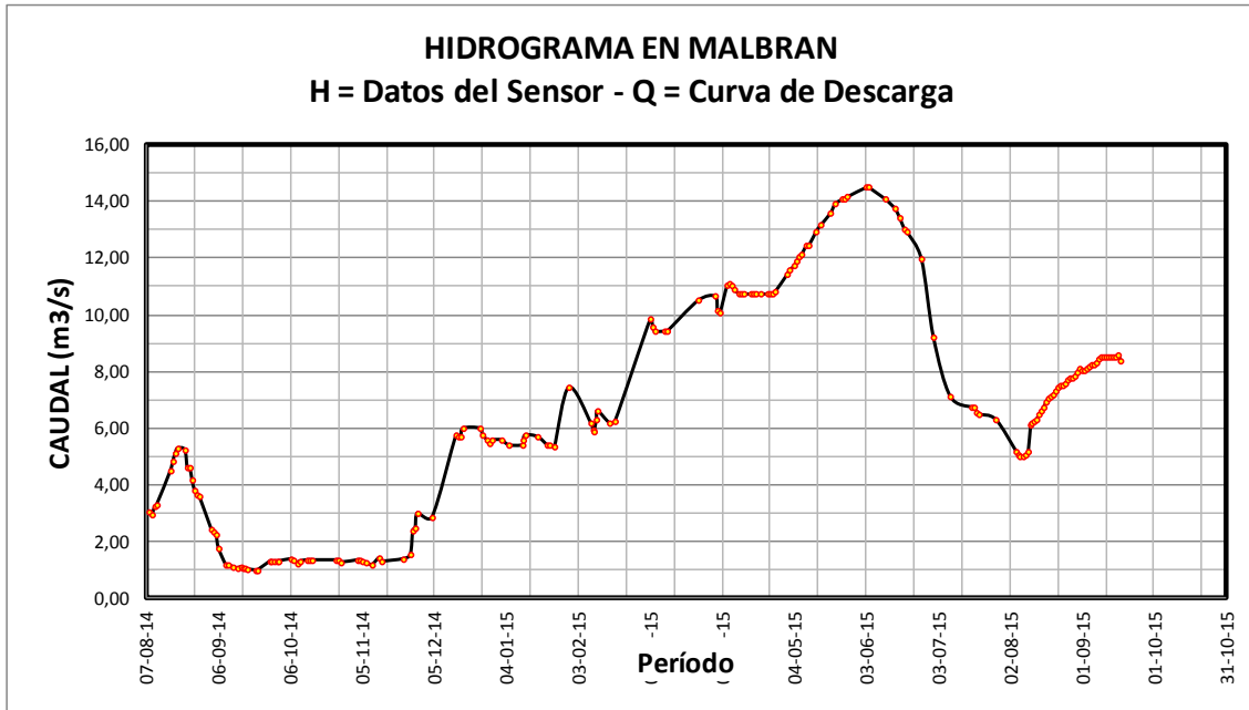
Gráfico de alturas registradas por el sensor y caudales calculados por la curva de descarga. Se presenta el período 08/08/2014 al 31/08/2015.
