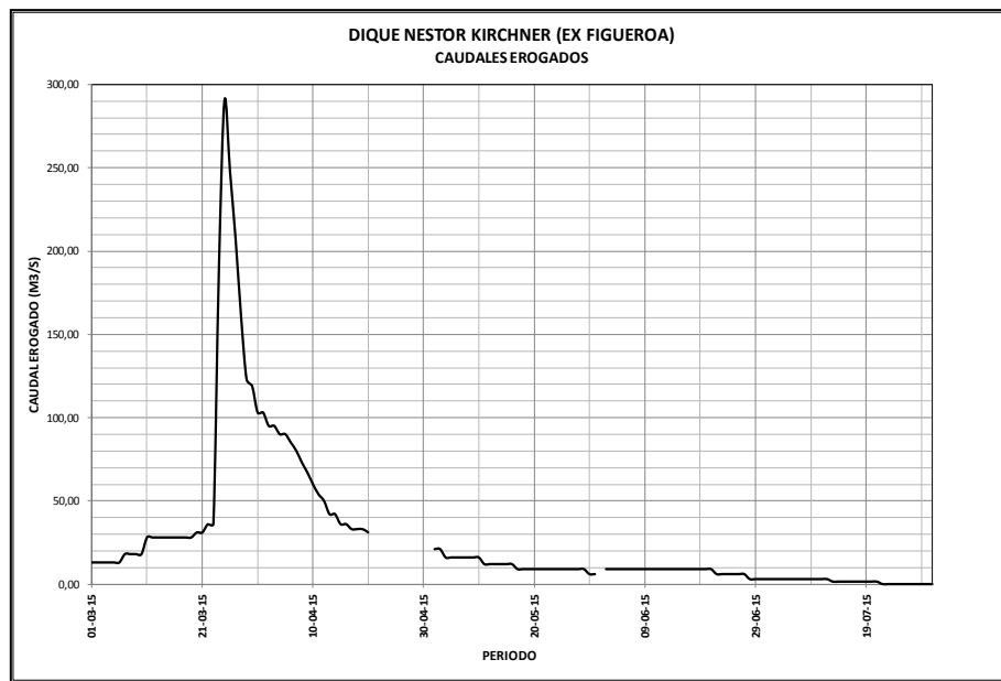
Caudal erogado por vertedero. Período 01/03/2015 – 31/07/2015
