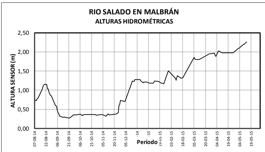
Alturas registradas por el sensor. Período 08/08/2014 al 31/05/2015.
