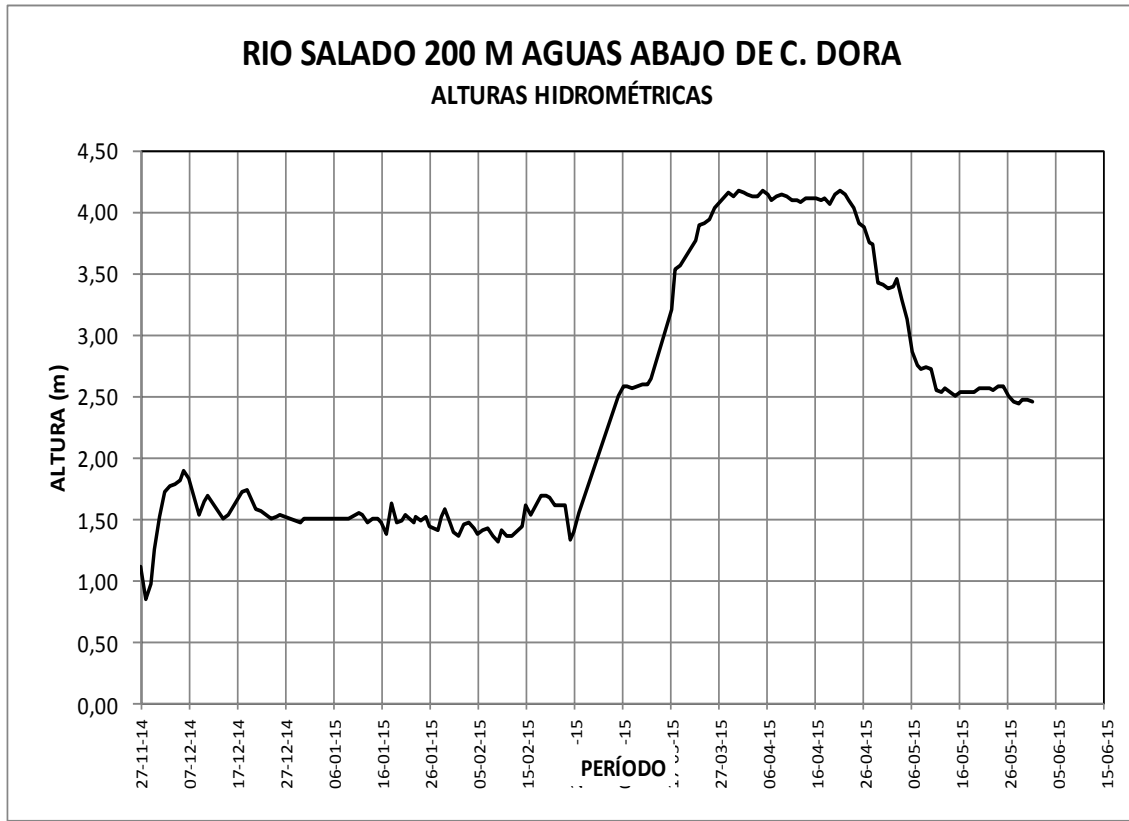
Alturas Hidrométricas 200 m aguas abajo C. Dora correspondientes al sensor de presión perteneciente al MASPyMA (Santa Fe). Período 27/11/2014 – 31/05/2015
