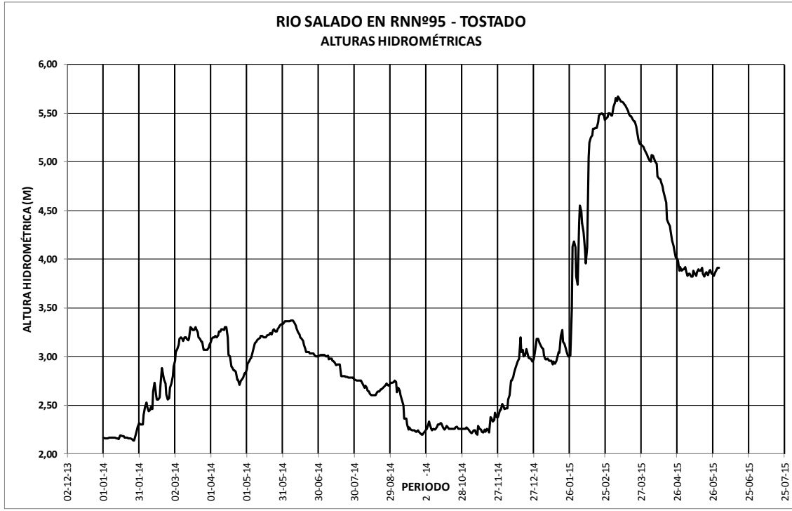
Alturas Hidrométricas período 01/01/2014 – 31/05/2015
