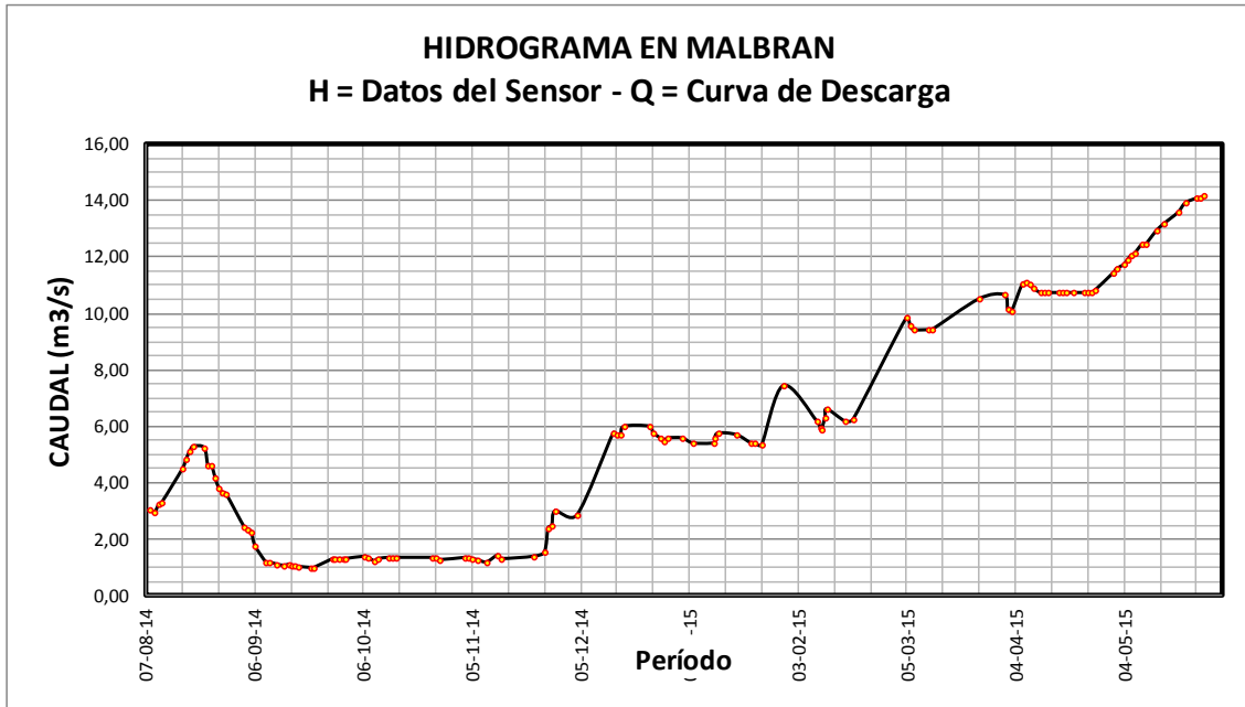
Hidrograma calculado con alturas registradas por el sensor y caudales calculados por la curva de descarga. Se presenta el período 08/08/2014 al 31/05/2015.
