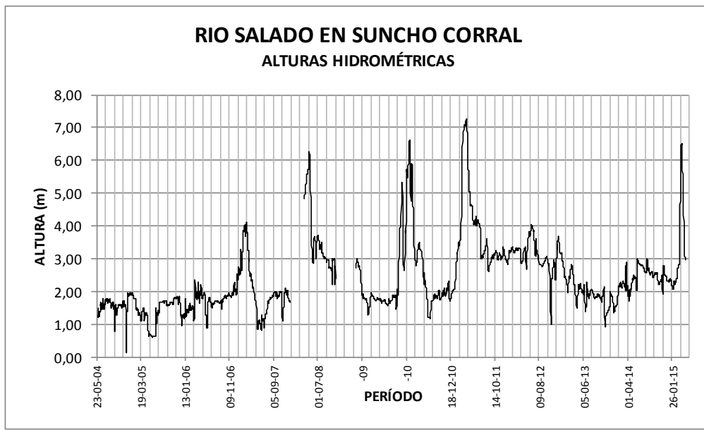
Alturas Hidrométricas pertenecientes a la BDI de la SSRHN – Período 30/05/2004 – 29/04/2015
