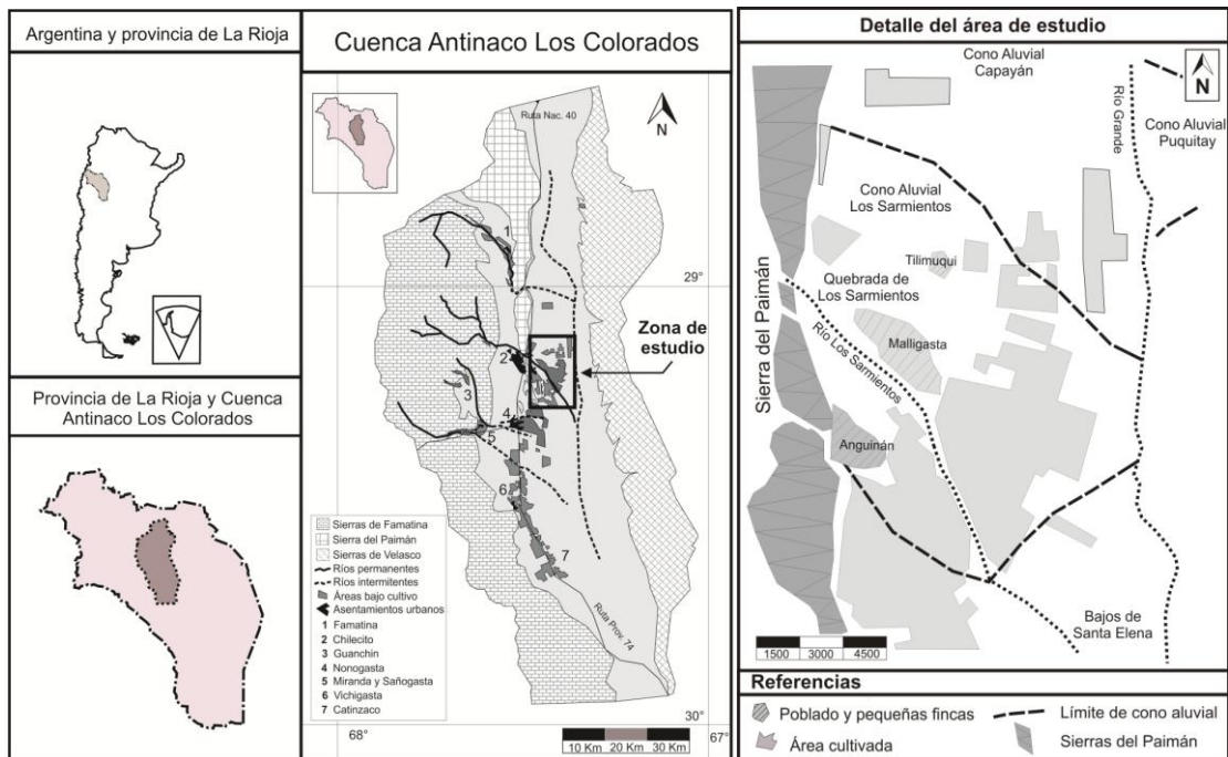
Figura 1. Área de estudio. Elaboración propia.
