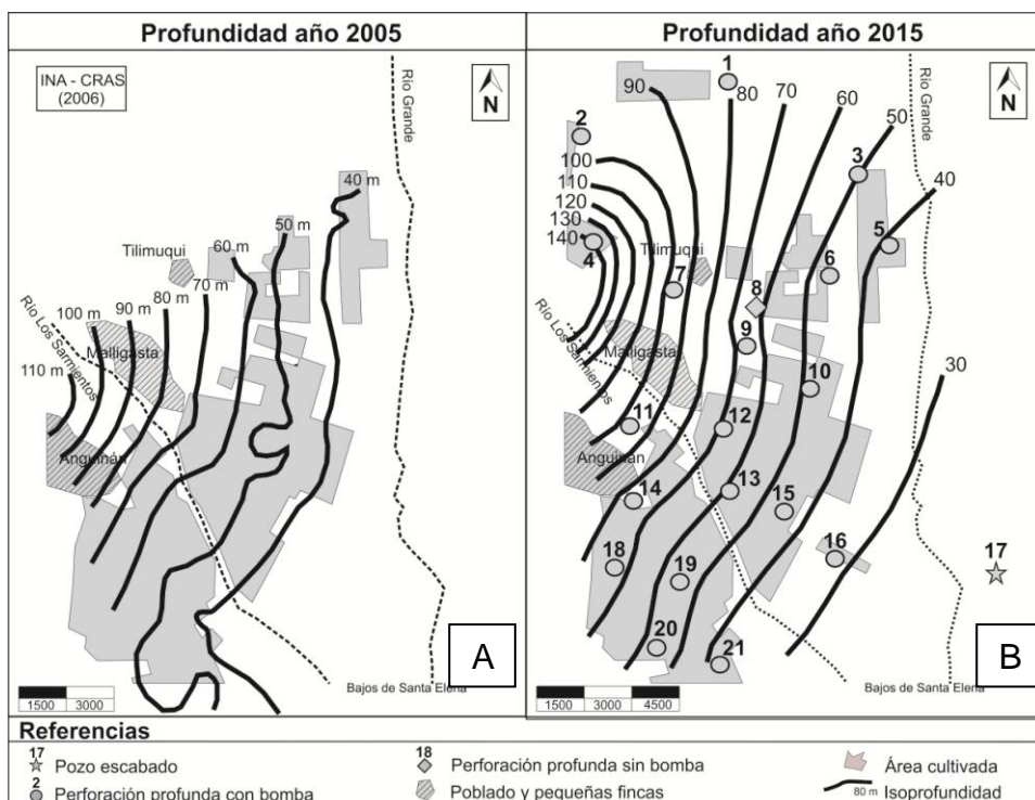
Figura 3. (A) Isoprofundidad al año 2005 (B). Isoprofundidad al año 2015. Elaboración propia.
