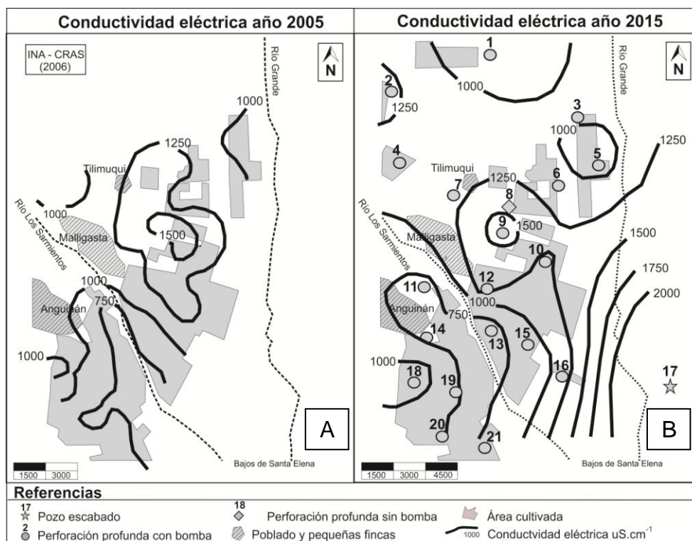
Figura 4. (A) Isoconductividad al año 2005 (B) Isoconductividad al año 2015. Elaboración propia.
