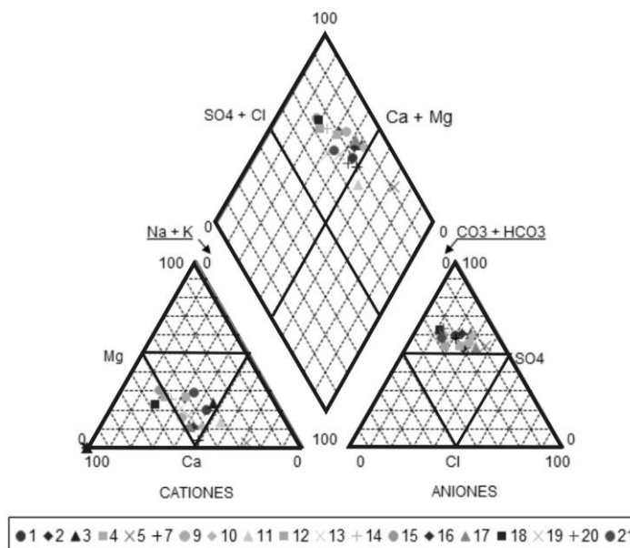
Figura 5. Diagrama de Piper e hidroquímica de las muestras. Elaboración propia.
