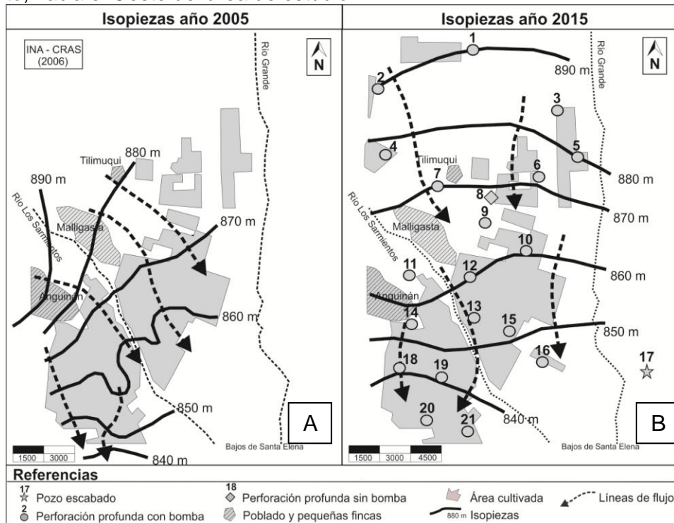
Figura 2. (A) Isopiezias año 2005 (B) Isopiezias 2015. Elaboración propia.
